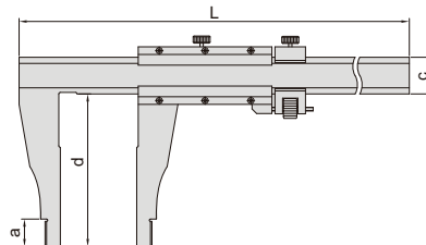
开式游尺(带螺钉)
